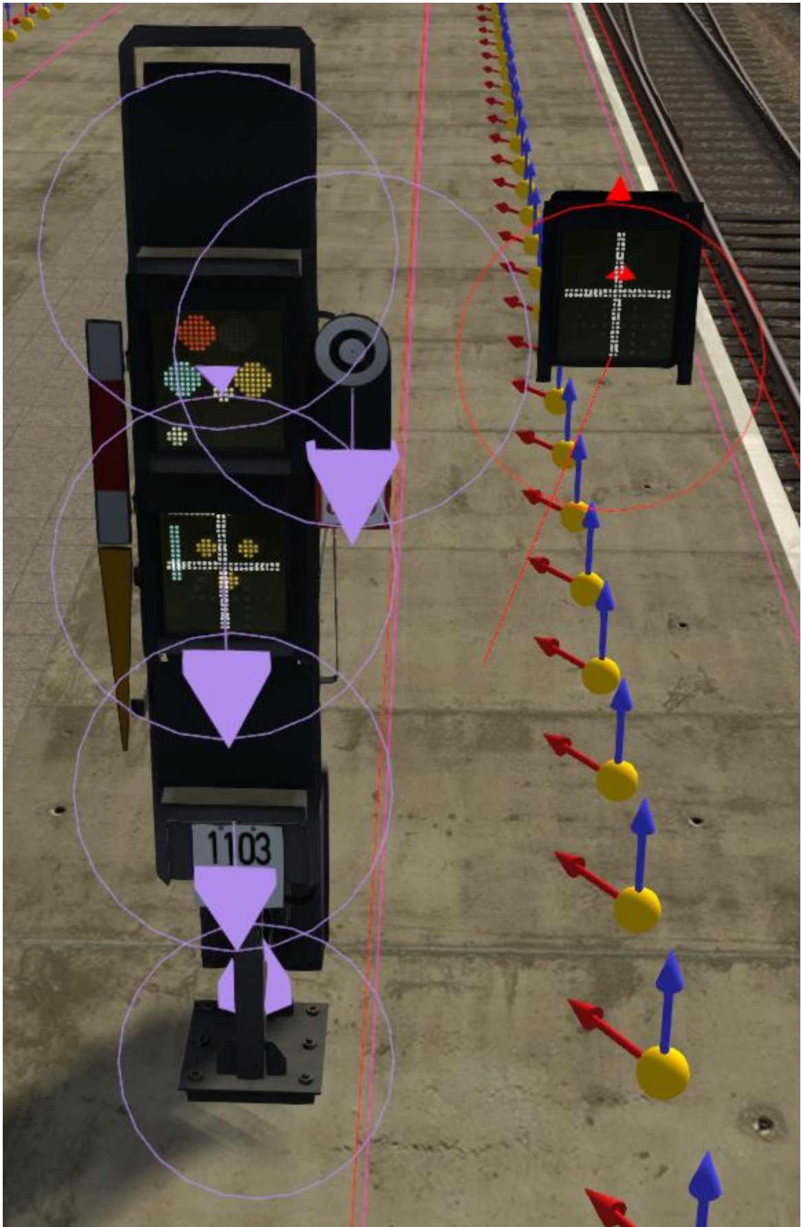
Abbildung 19 - Signal KS kSB MS 4x mit den vorhandenen Snapping Points
