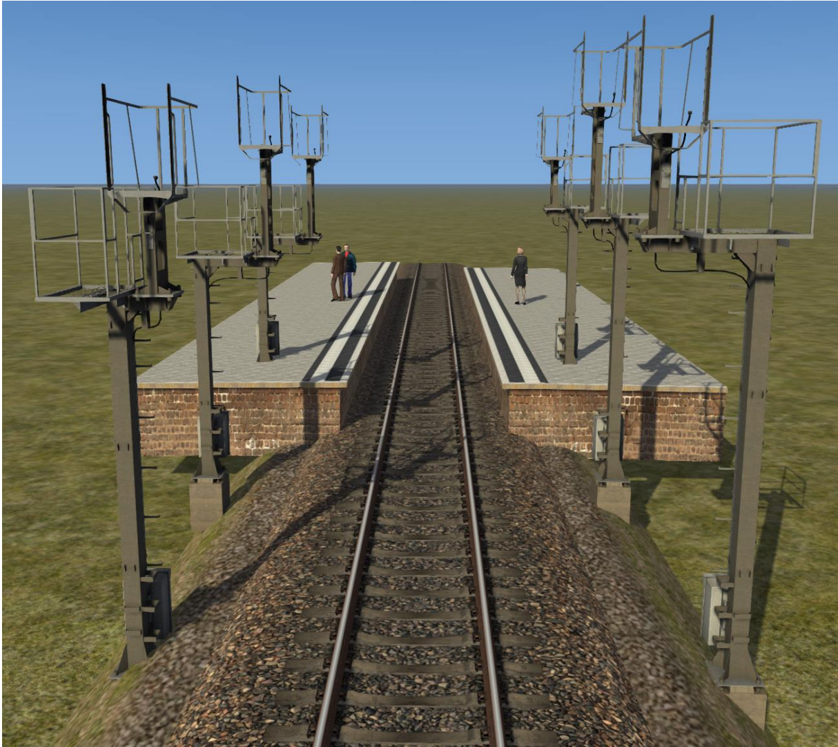
Abbildung 14 - Kombination der verschiedenen Auslegermasten
