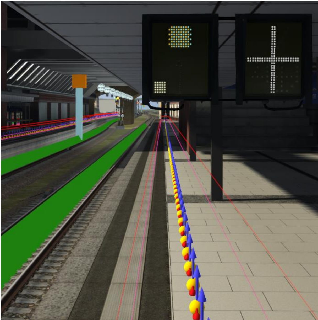
Abbildung 20 - Vorsignalwiederholer mit Zs 3v unterhalb vom Bahnsteigdach
